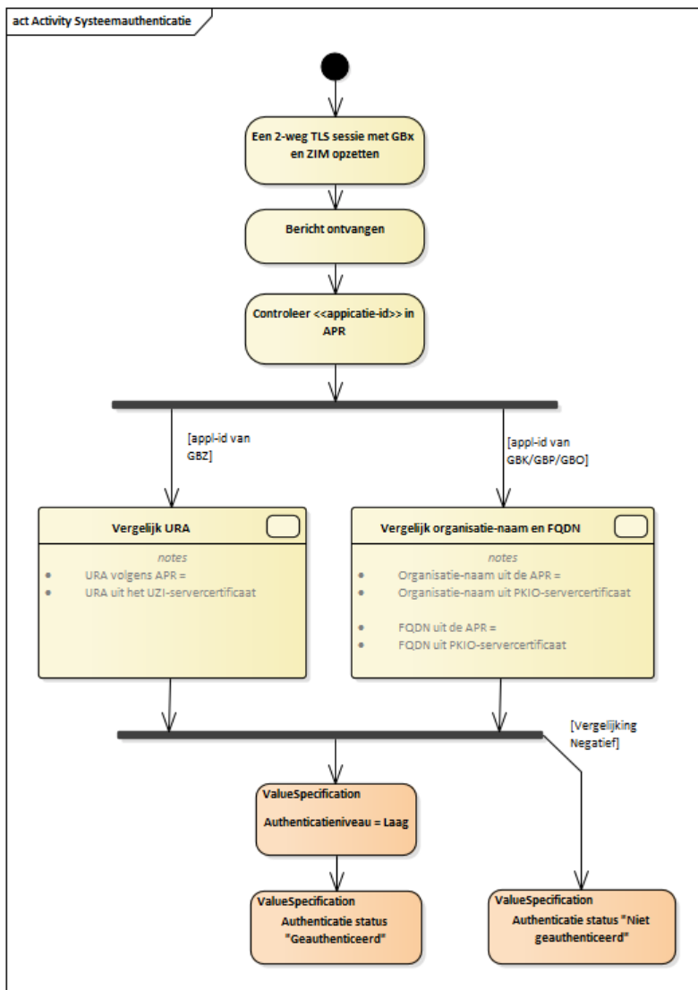
Figuur 2: Systeemauthenticatie
