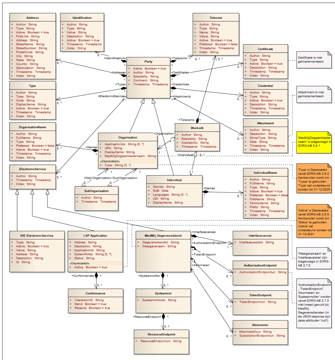
Figuur 1. Datamodel ZORG-AB 2.9.4
